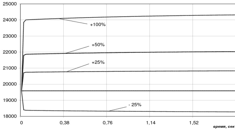
Рис. 2. Изменение значений \partial T / \partial r во времени при изменении расхода воды.
